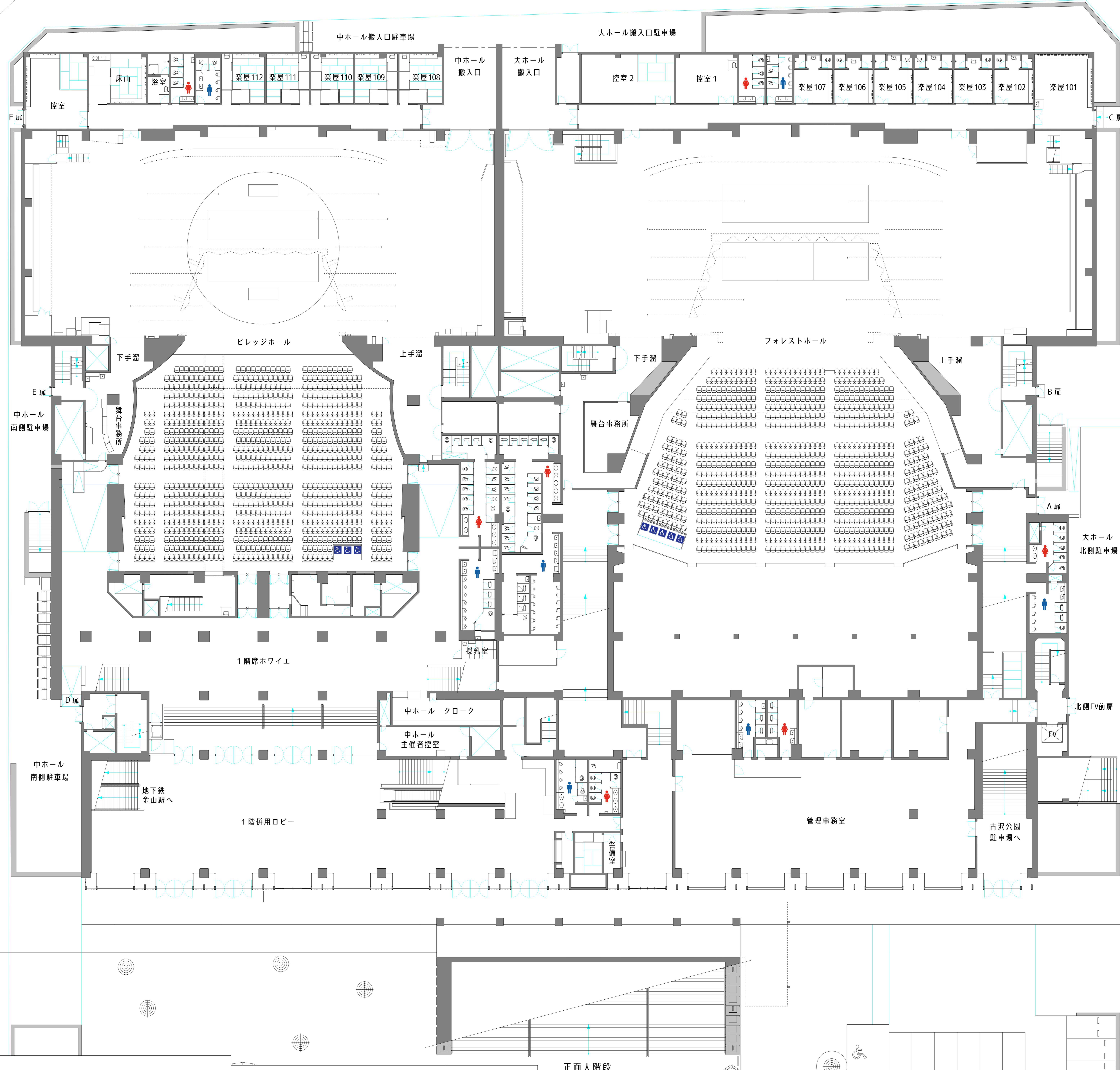
1階 平面図
