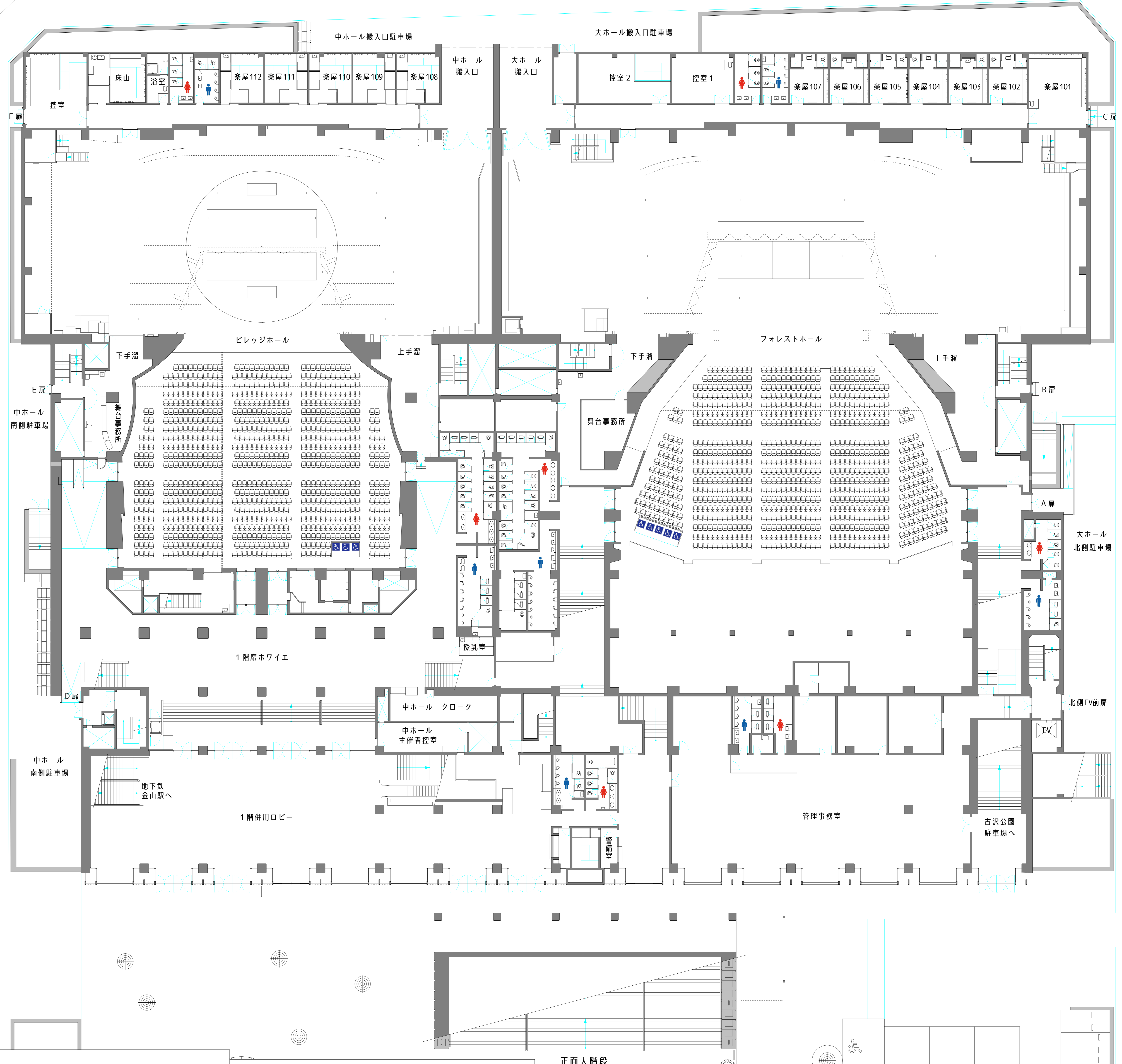
1階 平面図
